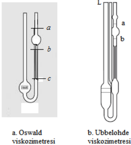
Şekil 3. Viskozite ölçümünde kullanılan iki ayrı viskozimetre
